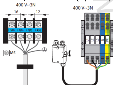
VNITŘNÍ JEDNOTKA
