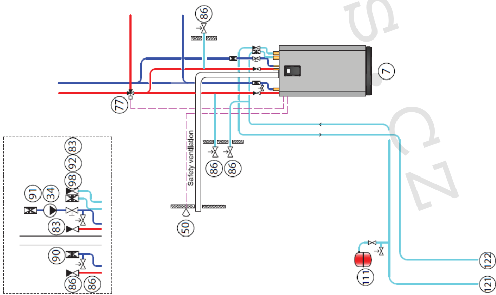
Mega E s HGW, bez oběhového čerpadla
