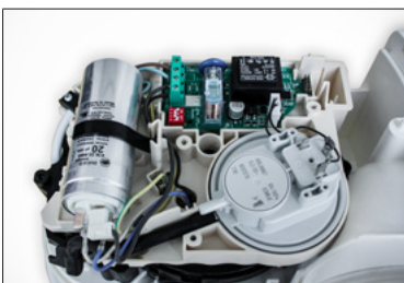
JEDNODUCHÝ PŘÍSTUP KU KONDENZÁTORU, TLAK. SPÍNAČU, EL. DOSKE
